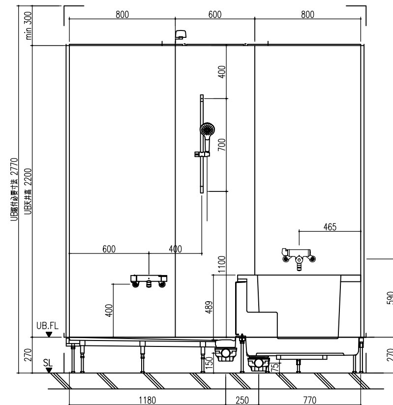
A 展開図
