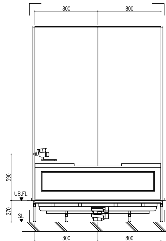
B 展開図
