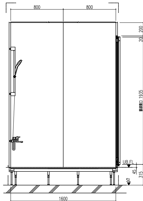
B 展開図
