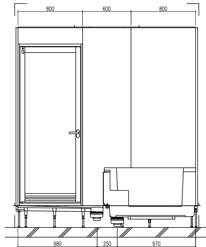
C 展開図
