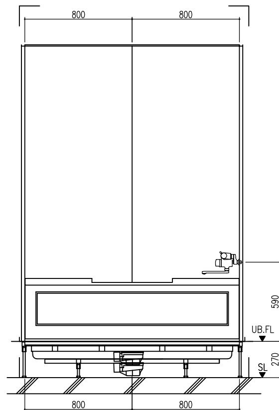
D 展開図
