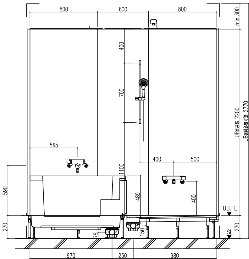
A 展開図
