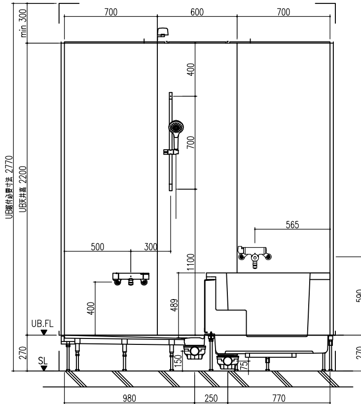
A 展開図
