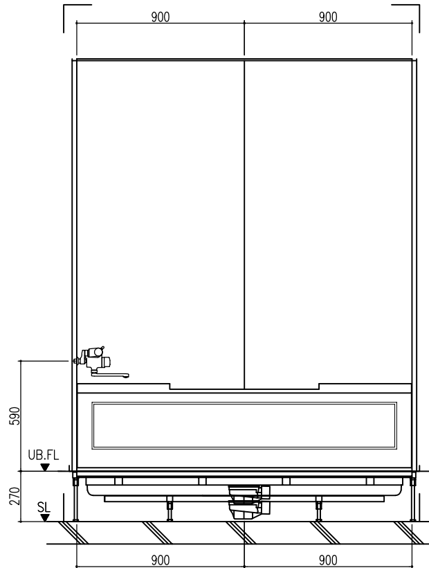
B 展開図
