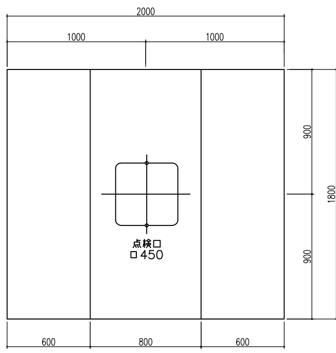
天井伏図
