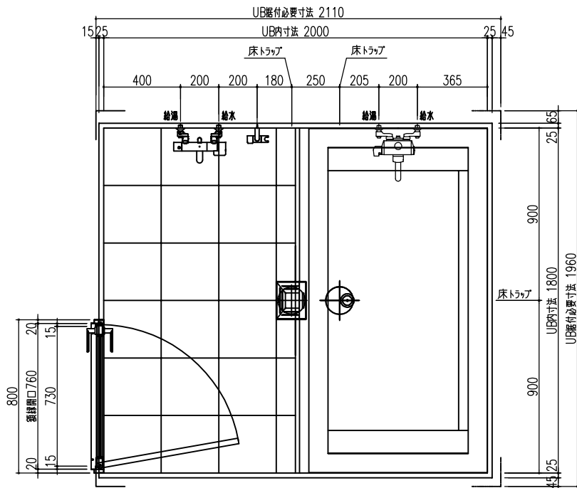
平面図
