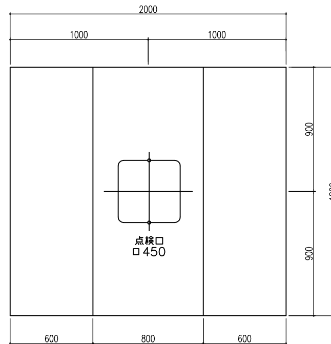
天井伏凶
