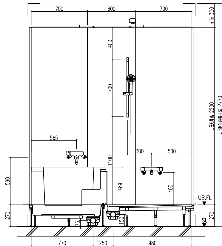
A 展開図
