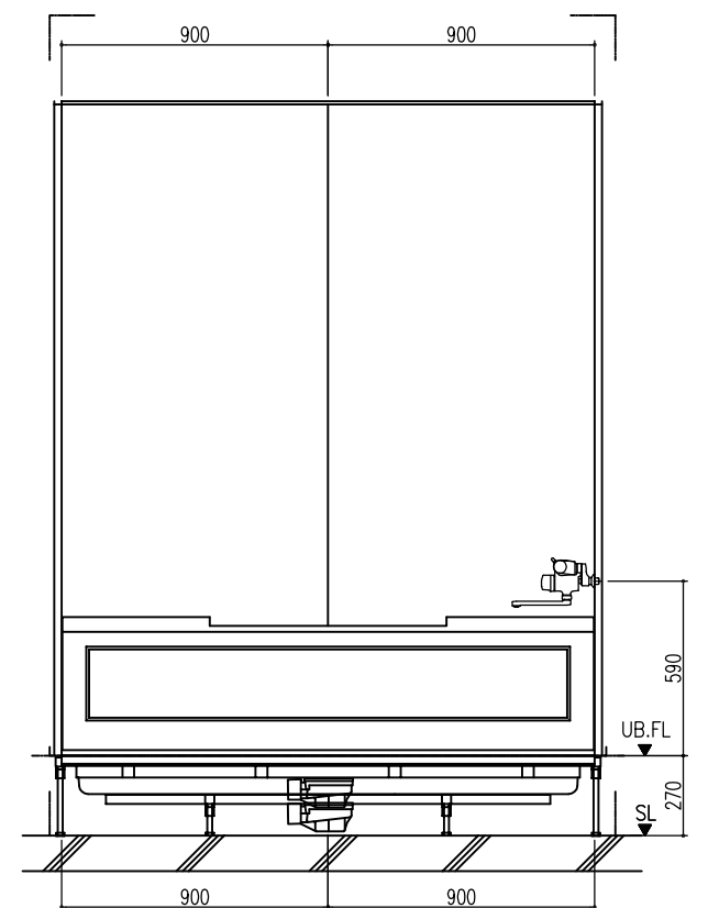
D 展開図
