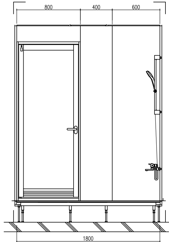
D 展開図
