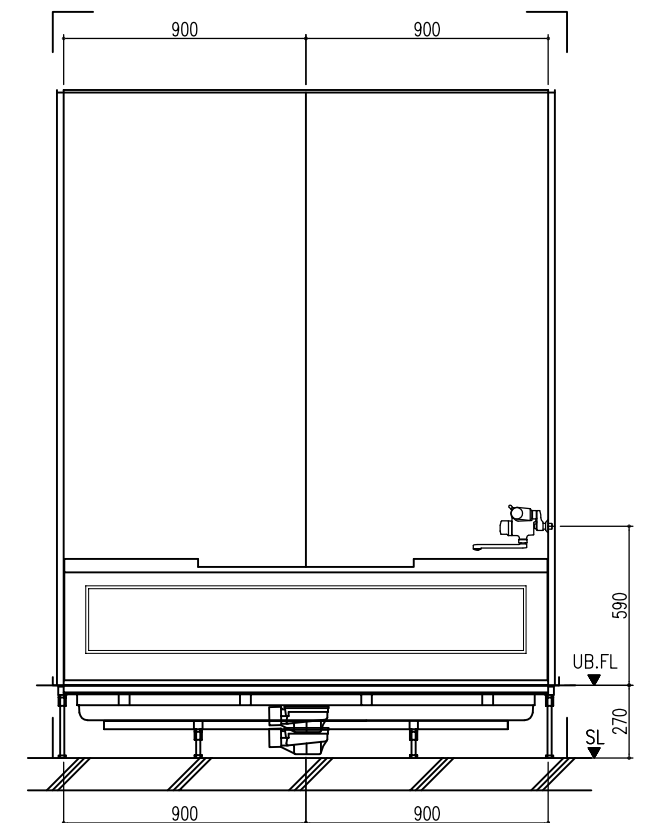
D 展開図
