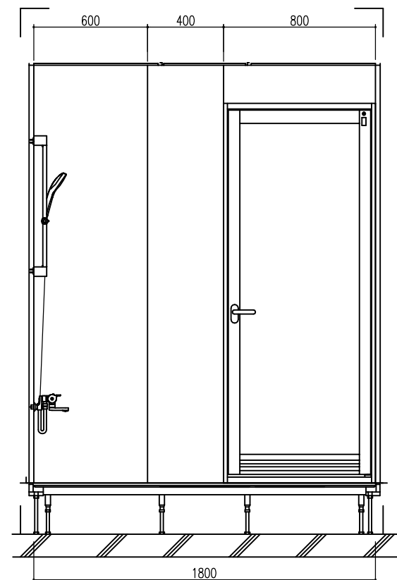
B 展開図
