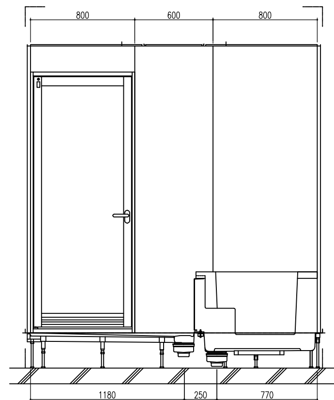
C 展開図
