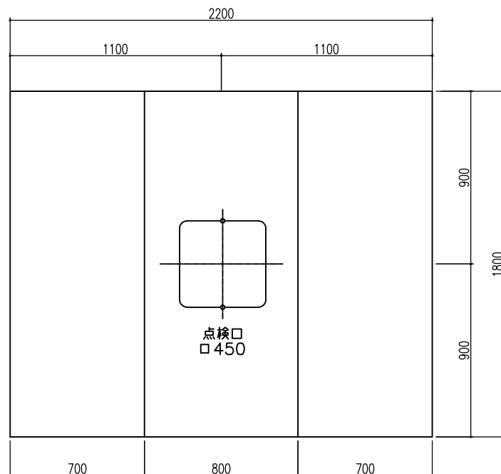
天井伏図
