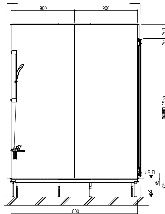
B 展開図
