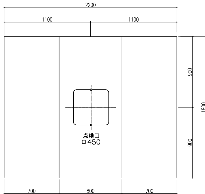
天井伏図
