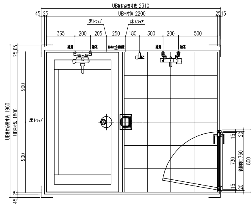
平面図
