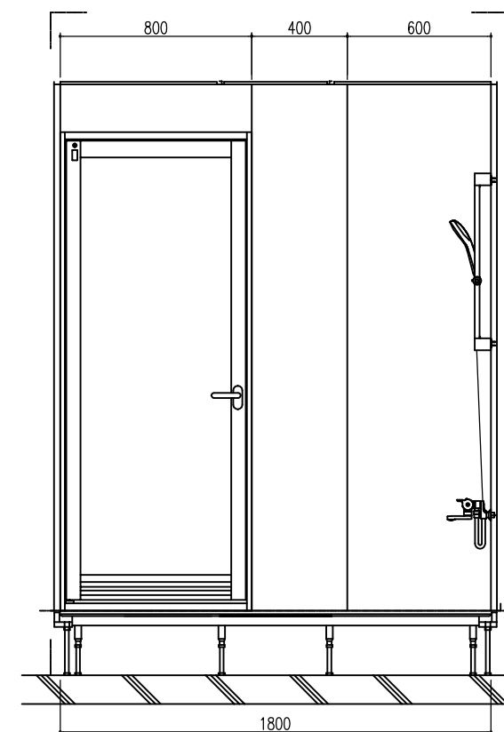
D 展開図
