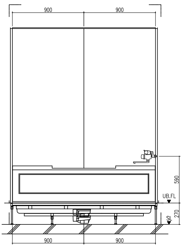
D 展開図
