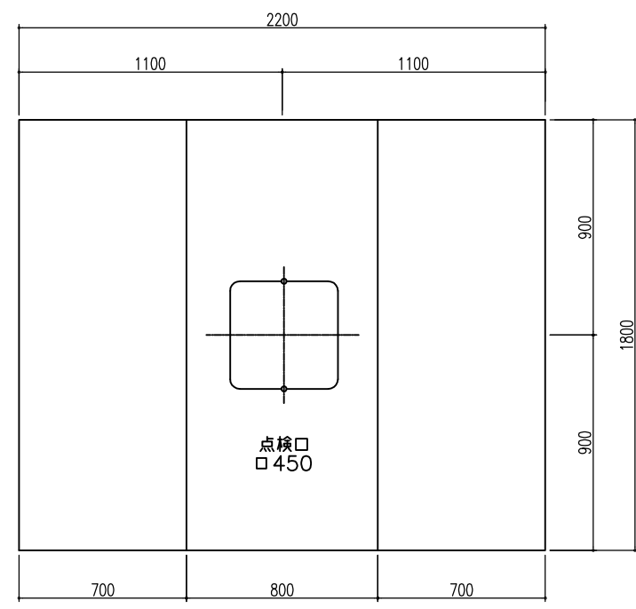
天井伏図
