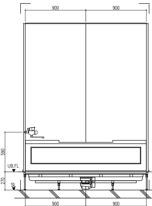
B 展開図
