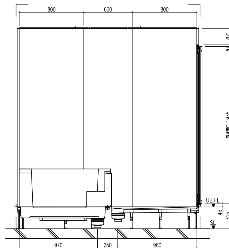
C 展開図
