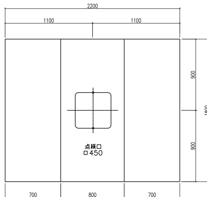
天井伏図
