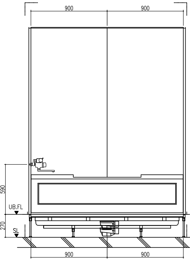
B 展開図
