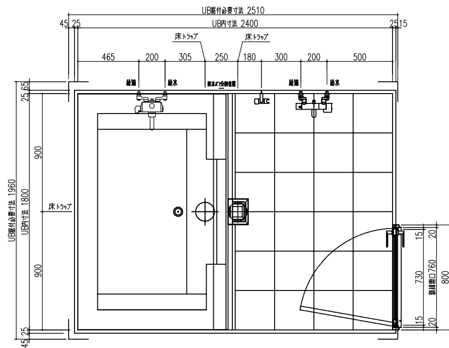
平面図
