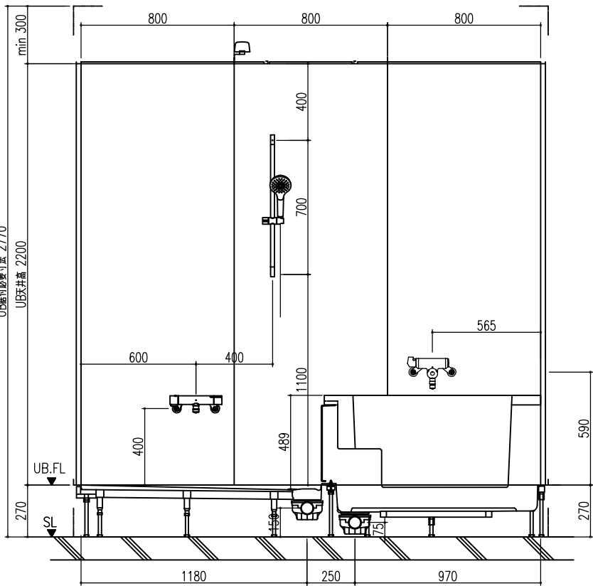
A 展開図
