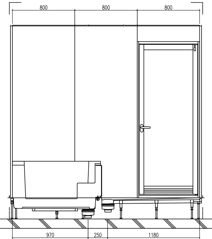
C 展開図
