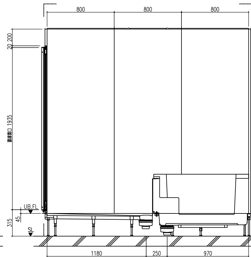
C 展開図
