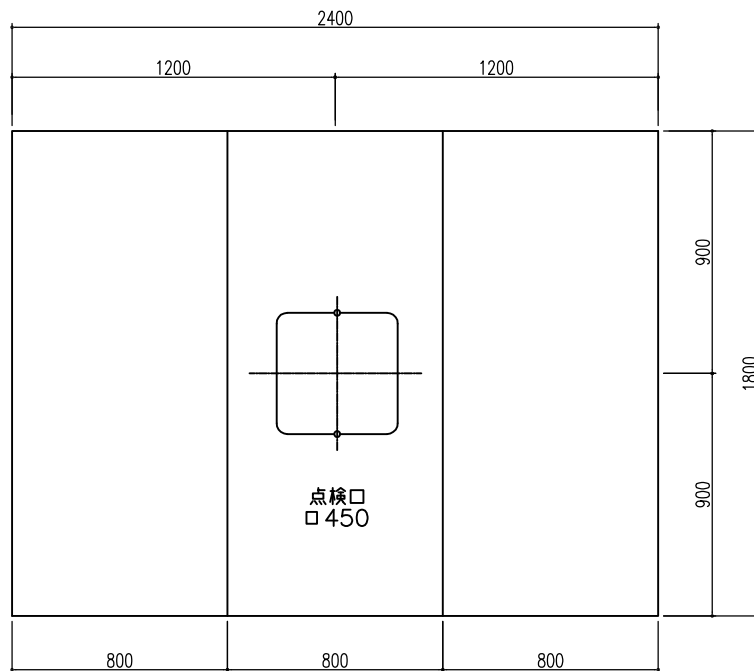
天井伏図
