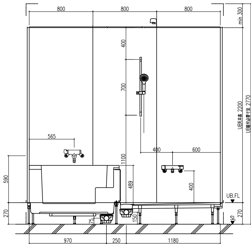
A 展開図
