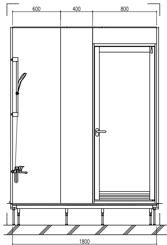
B 展開図
