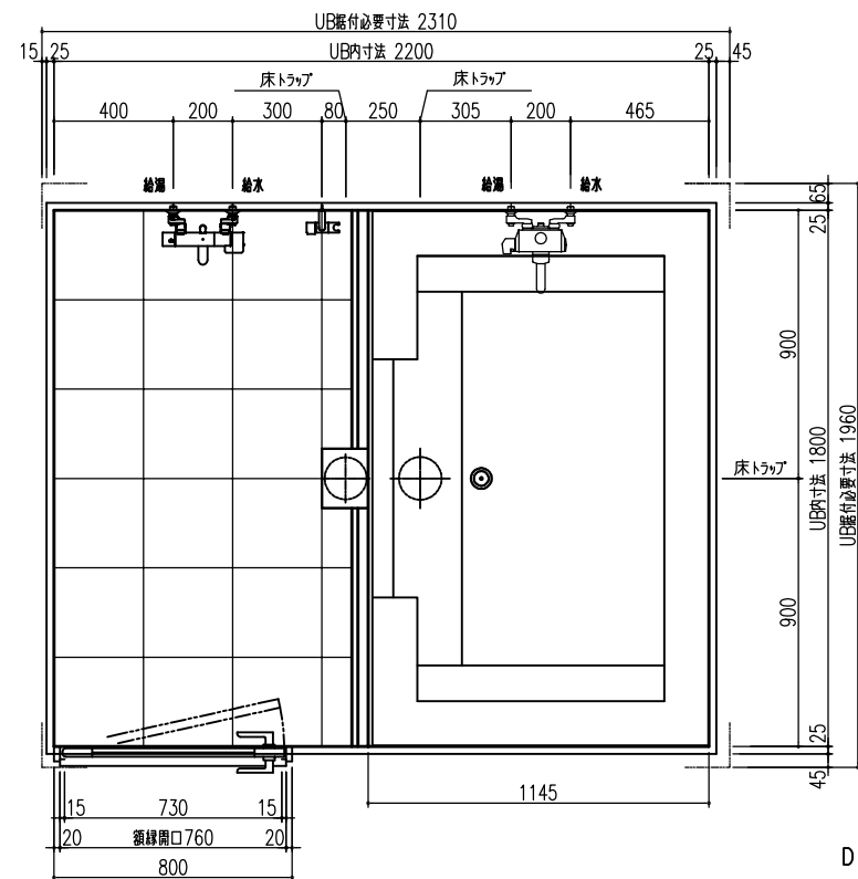
平面図
